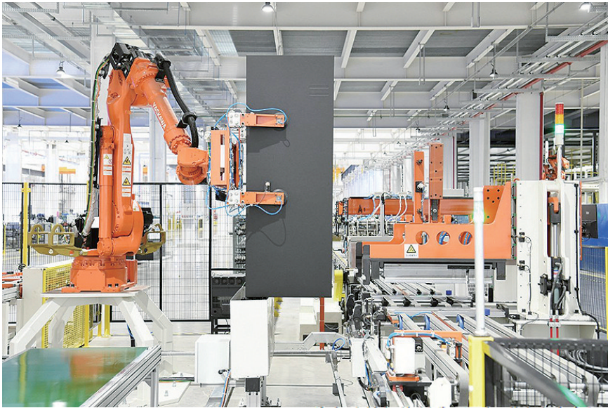
海尔冰箱智能制造项目（一期）生产车间。
