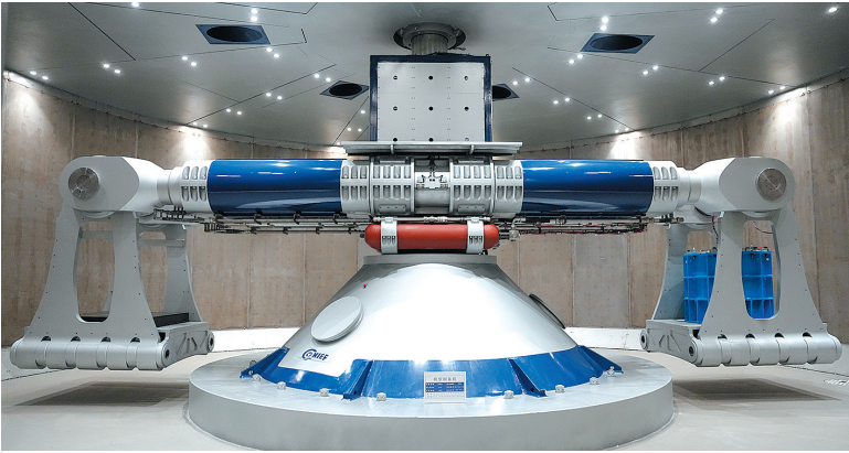
■9月29日拍摄的超重力离心模拟与实验装置启动的首台离心机主机。新华社照片
