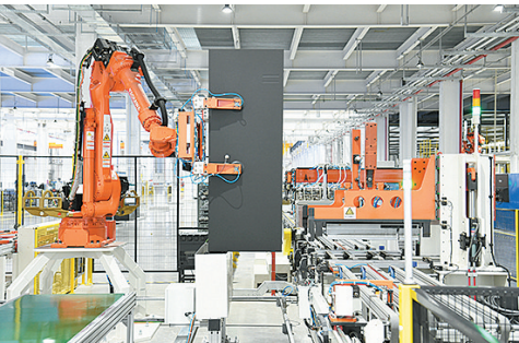
海尔卡奥斯工业互联网生态园冰箱智能制造(一期)项目生产线。
