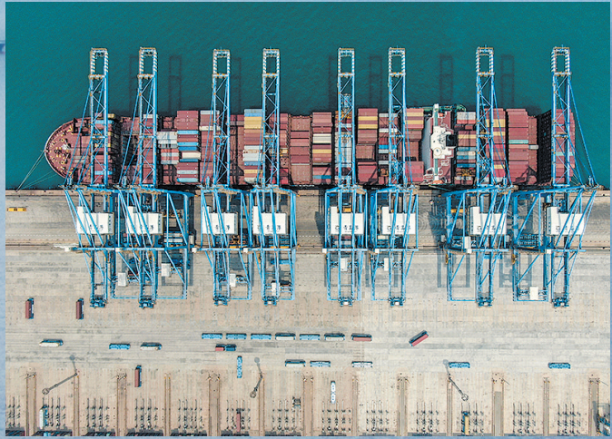
■青岛港全自动化码头让码头作业更快捷、更精准、更智能。 赵健鹏 摄
