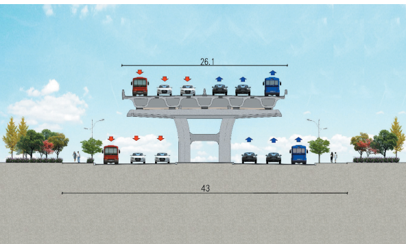
■高架标准段横断面示意图。
